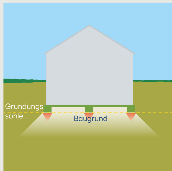
Nach Bauwerkserstellung: kleine Fläche, große Sohlspannung, kleine Tiefenwirkung
