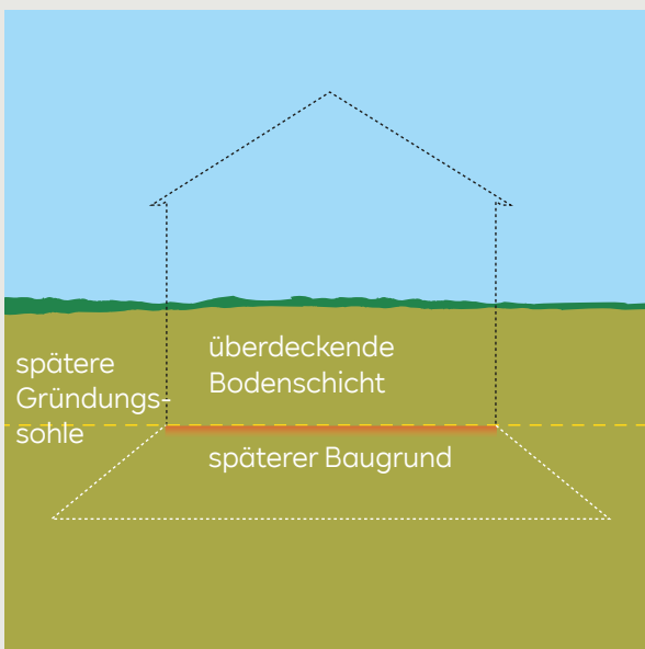
Vor Baubeginn: große Fläche, kleine Sohlspannung, große Tiefenwirkung
